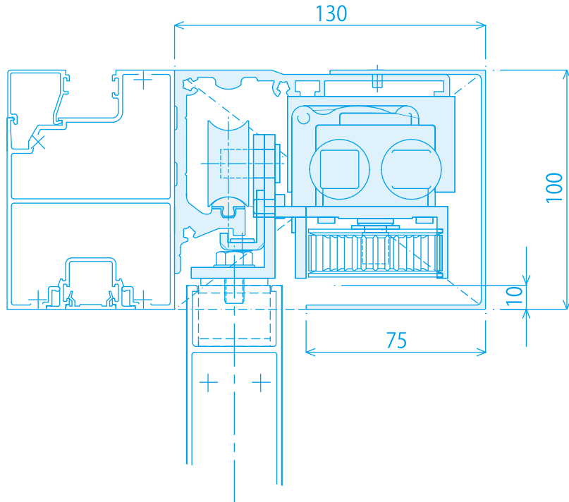
縦断面図 JA-100
