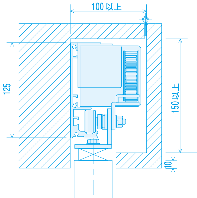
縦断面図 UN-150WD
