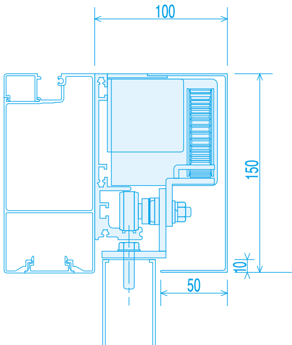
縦断面図 UN-150
