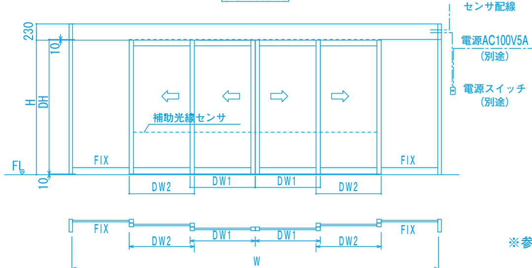
点検口側観図
