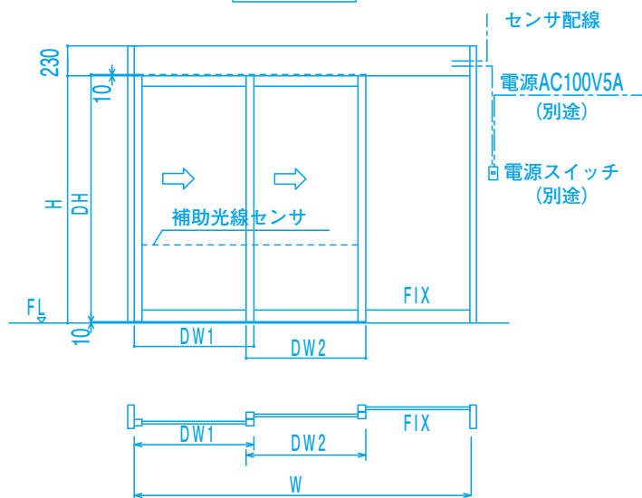
点検口側観図
