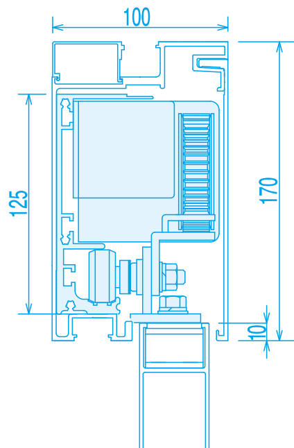
縦断面図
